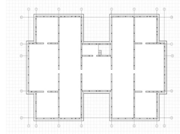
План третьего уровня блоков
