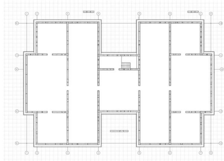
План фундамента
