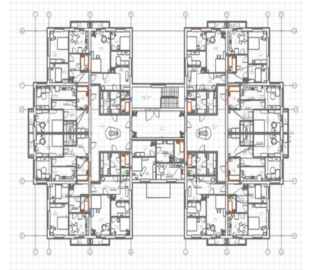
План последующих этажей (Совмещённый с АР)
