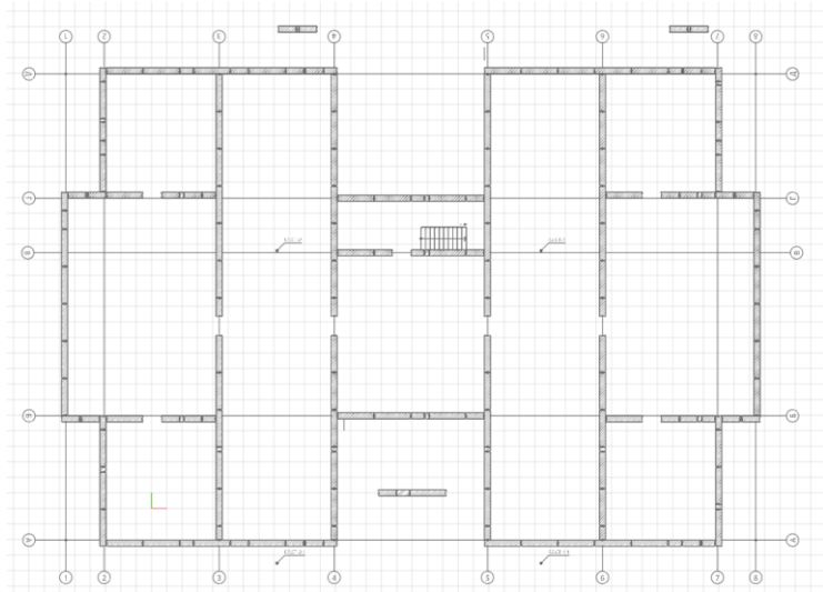
План второго уровня блоков
