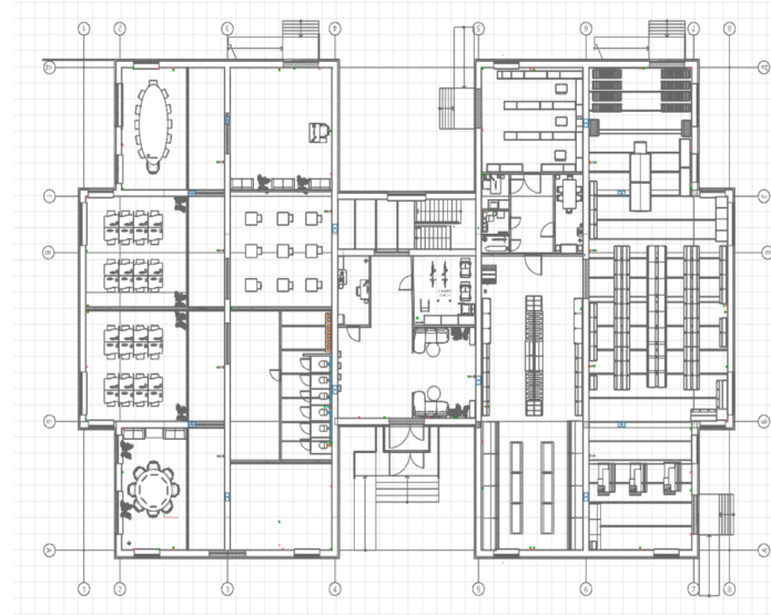
План первого этажа (Совмещённый с АР)
