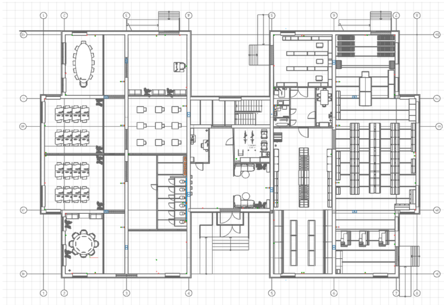
Вентиляционные сети
