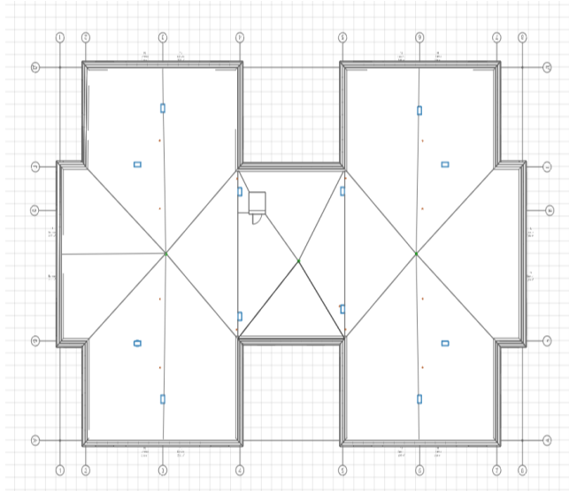
План крыши
